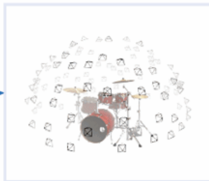
NeRF обучение
